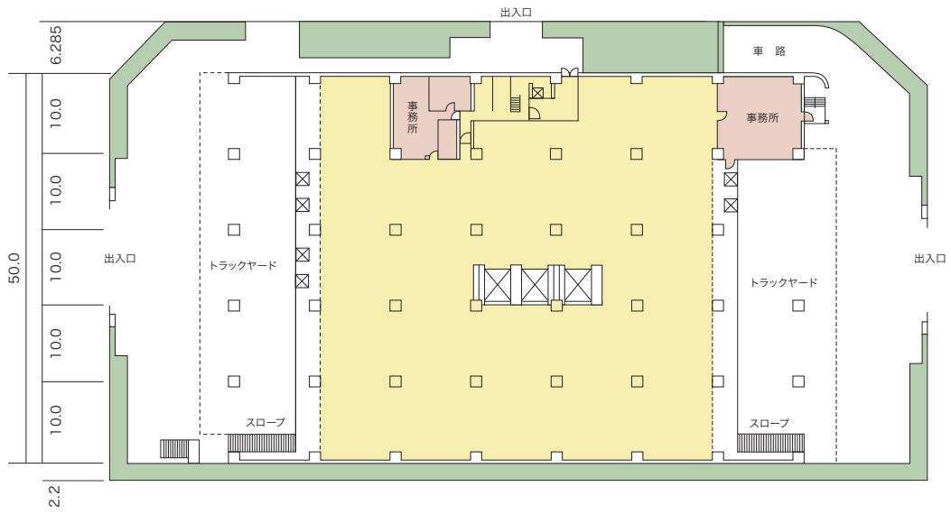
1階平面図
