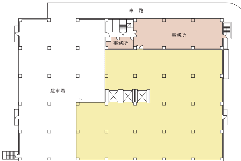
2階平面図
