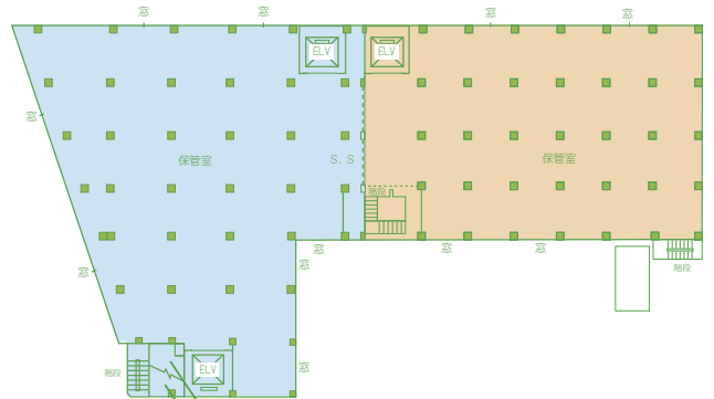
新館3階/旧館2階 新館4階/旧館3階 平面図
