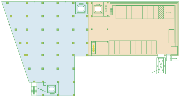
新館5階/旧館R階平面図
