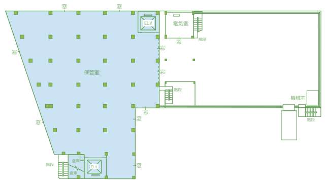
新館6階平面図
