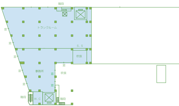
新館2階平面図
